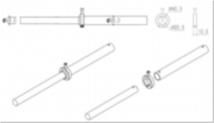
（实心冷轧圆钢+铝合金联轴器+冷轧圆管连接示意图，仅供参考）
