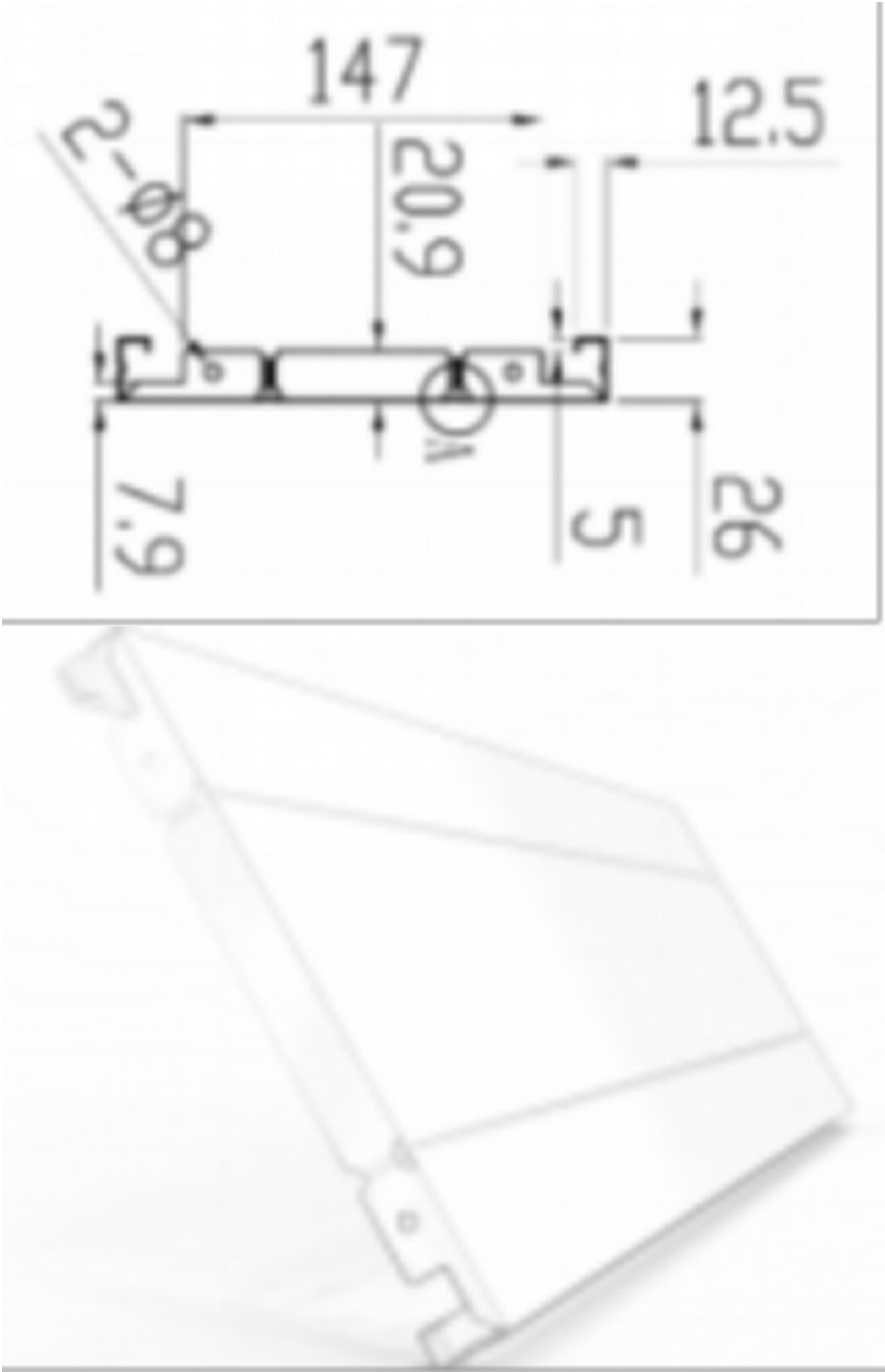
（搁板示意图，仅供参考）
